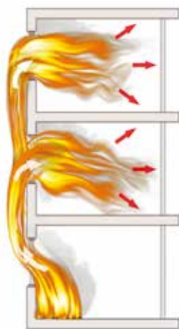
(Propagazione dell'incendio attraverso la facciata)
